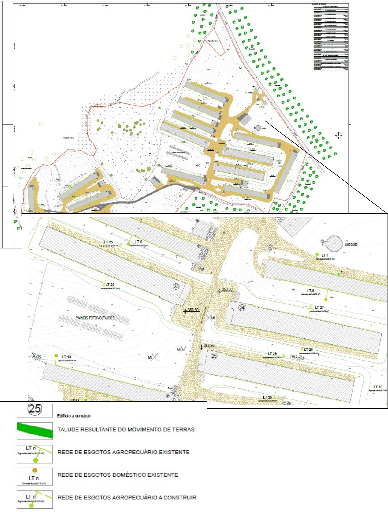
Cartografia 6 - Planta do projeto, com sinalização das infraestruturas de esgotos a construir.
